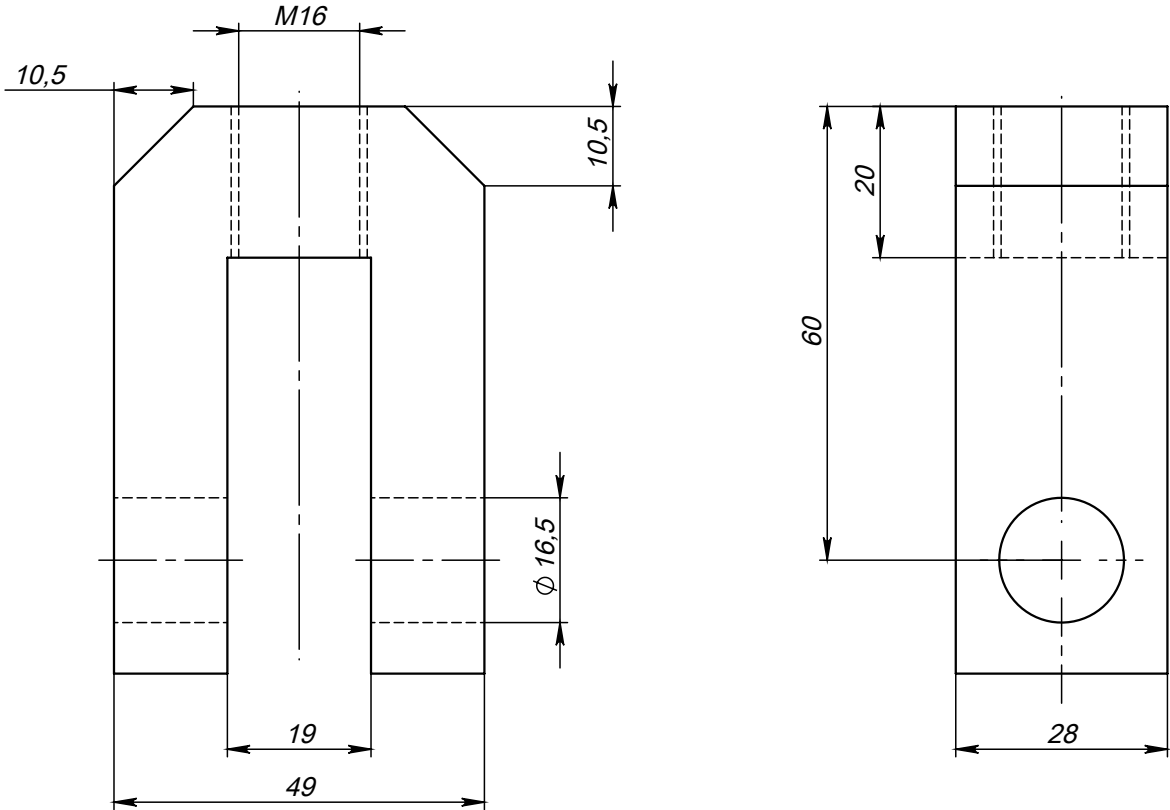
Поз. 1 (Вилка)
