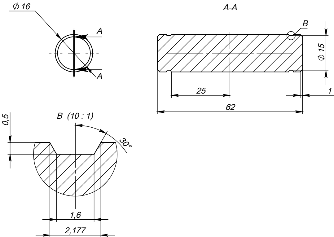
Поз. 2 (Стержень)
